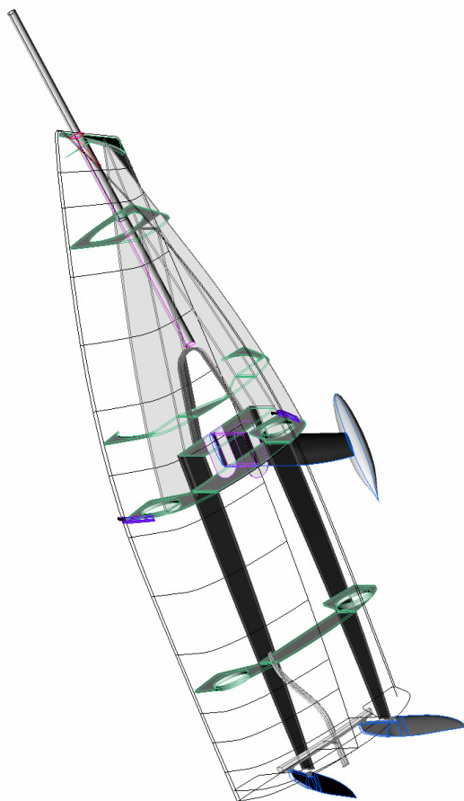
Strukturtegnning af Ternen, der bl.a. viser kølbrønd, bovspryd og mandehuller.
